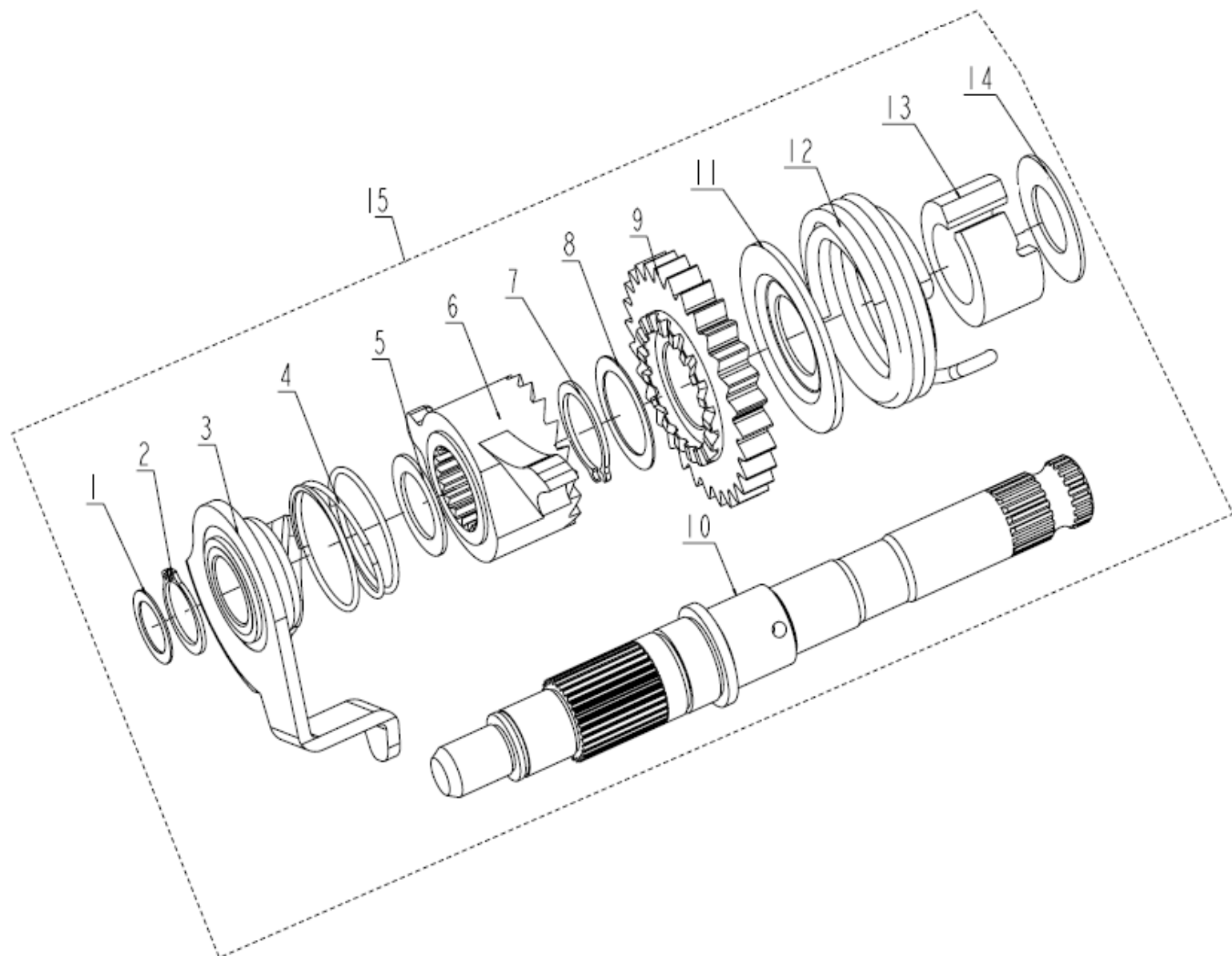
E12. 启动轴组合 KICK STARTER ASSY
