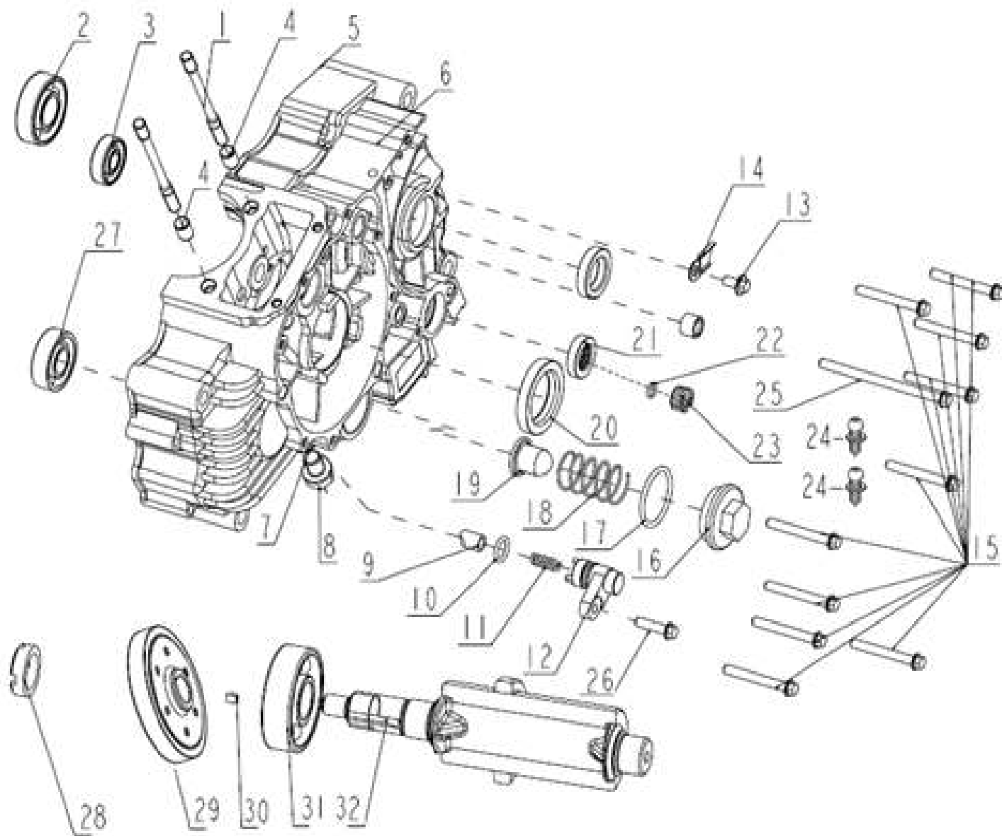
E14.左曲轴箱分总成 LEFT CRANKCASE ASSY
