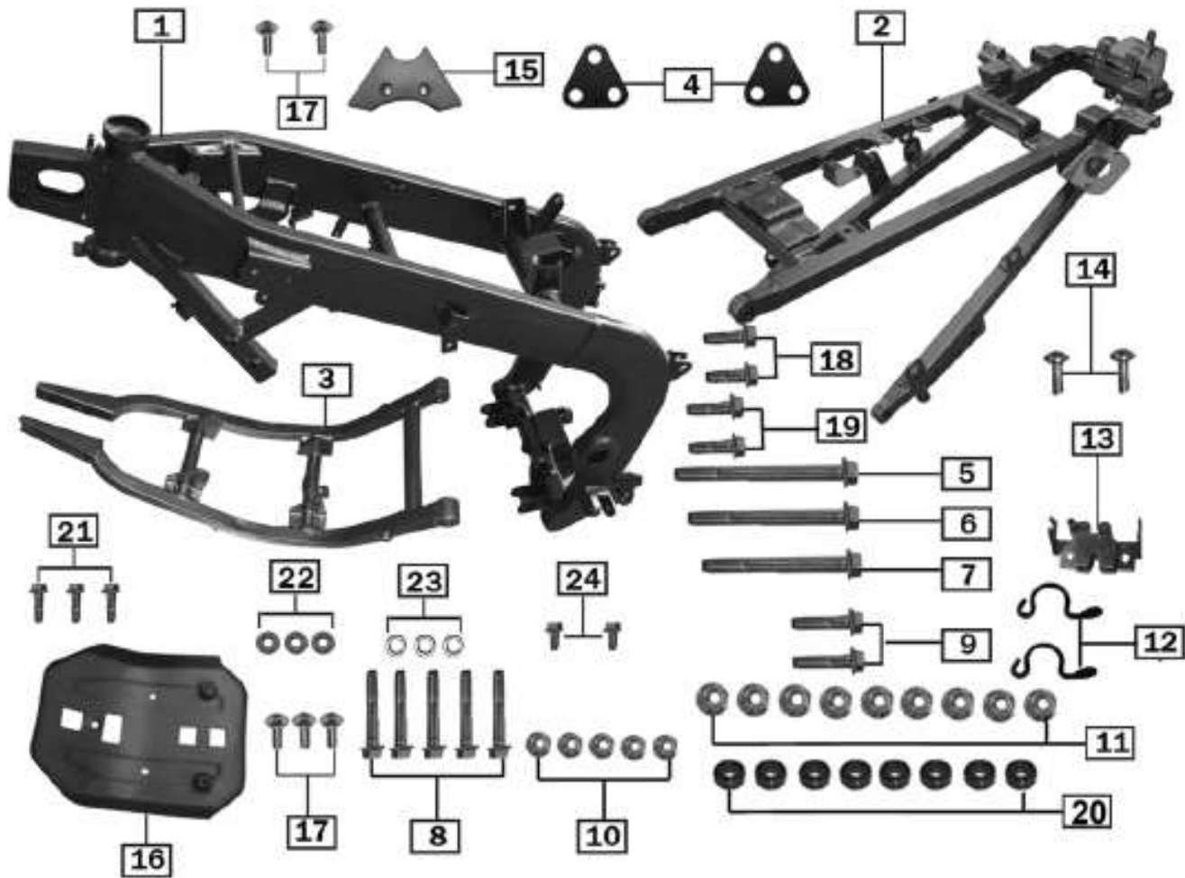
车架 frame
