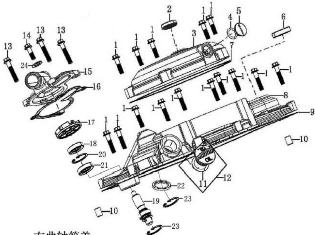
右曲轴箱盖
