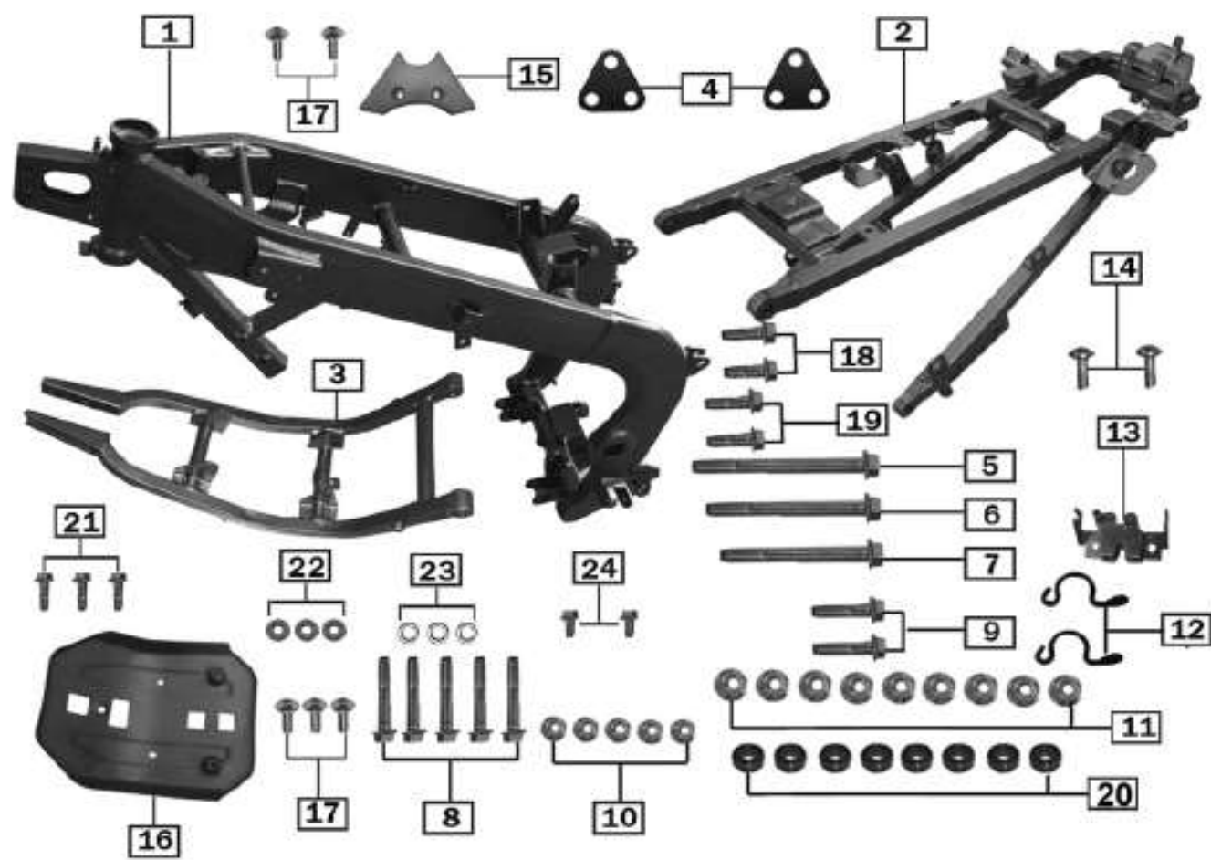
车架 frame
