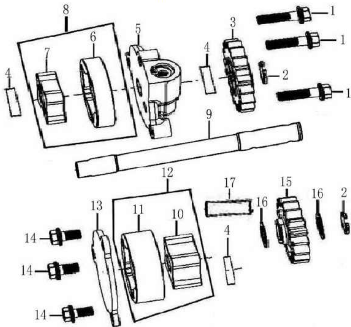
机油泵部件 OIL PUMP
