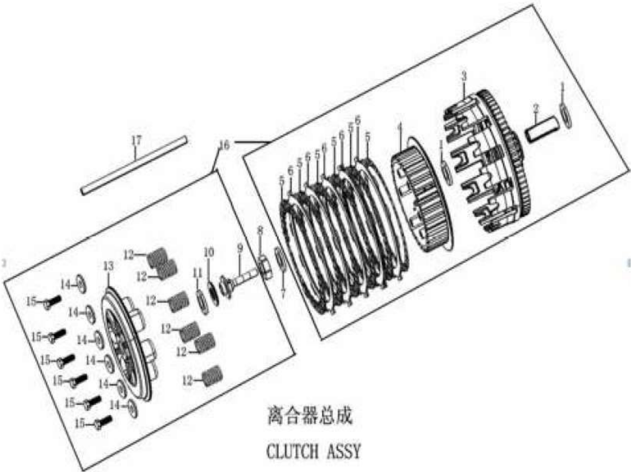
离合器总成 CLUTCH ASSY
