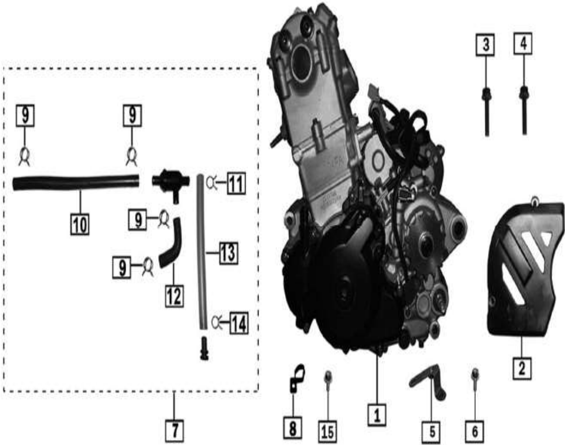
发动机ENGINE
