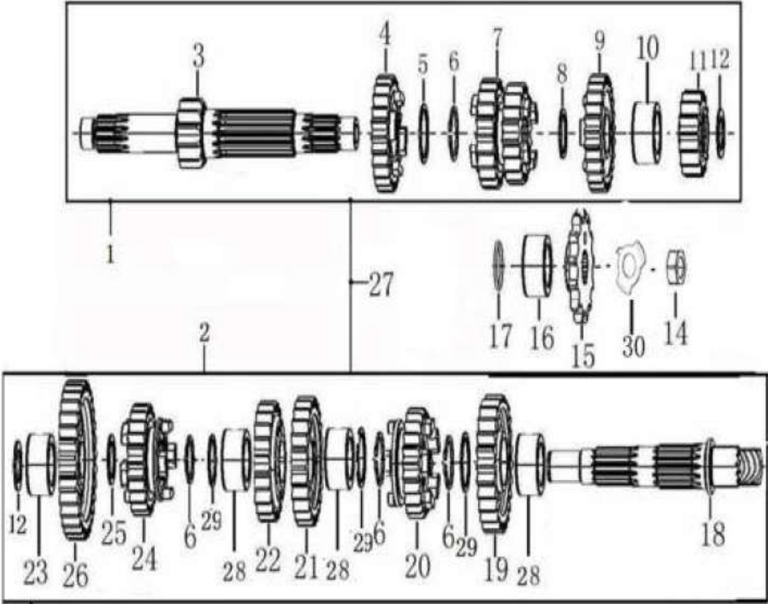
主副轴组合 TRANSMISSION MAIN,COUNTER SHAFT
